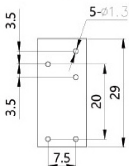
安装尺寸
